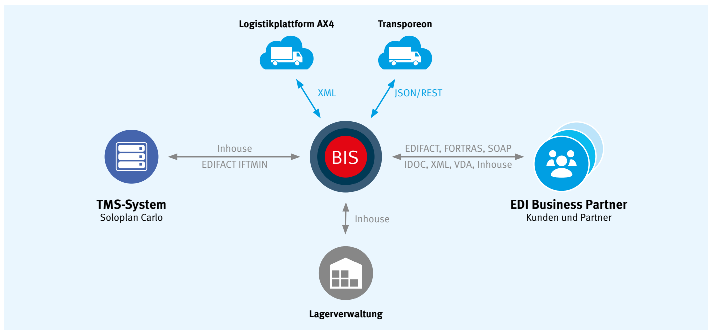
Abb. 1: Vernetzung der HAAF-Logistikanwendungen über die SEEBURGER BIS-Plattform
